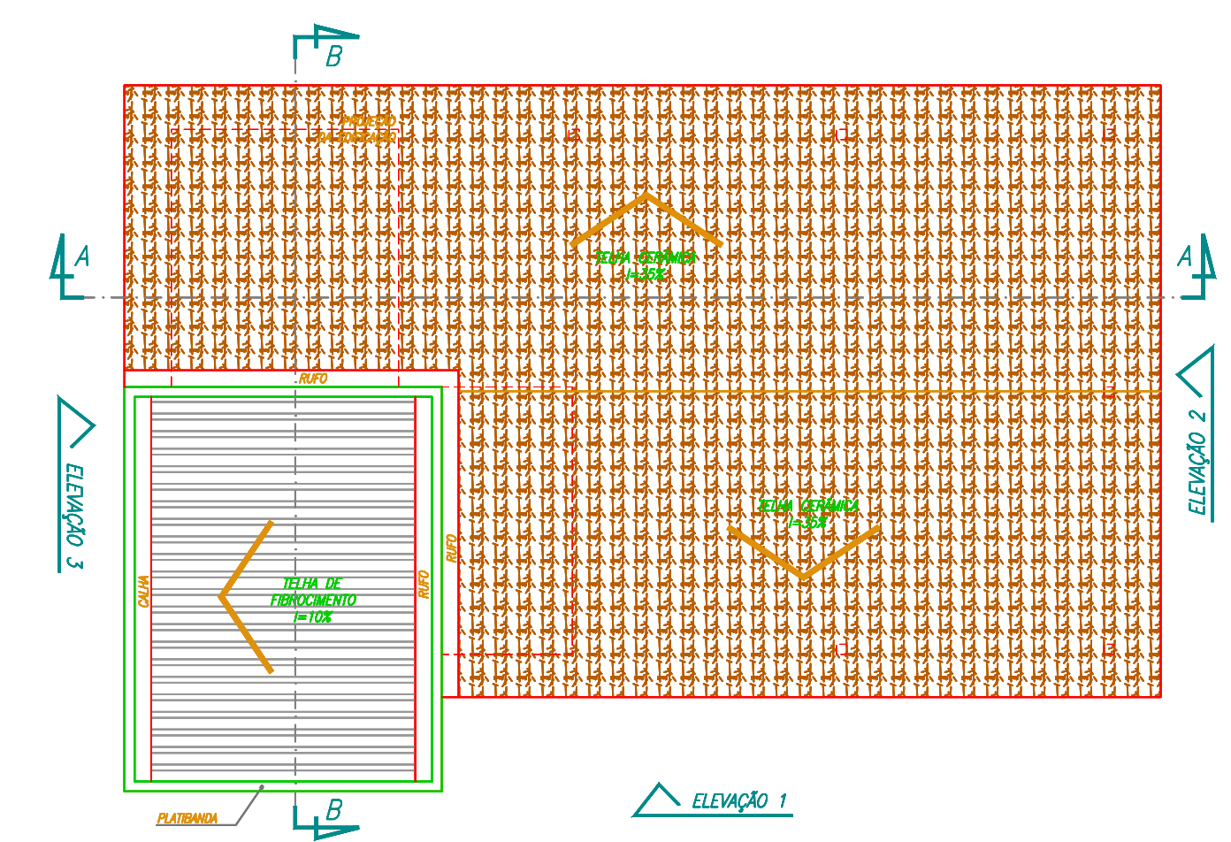
PLANTA DE COBERTURA ESC. 1:100
