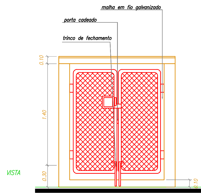
DETALHE DA CENTRAL GLP ESC. 1:25
