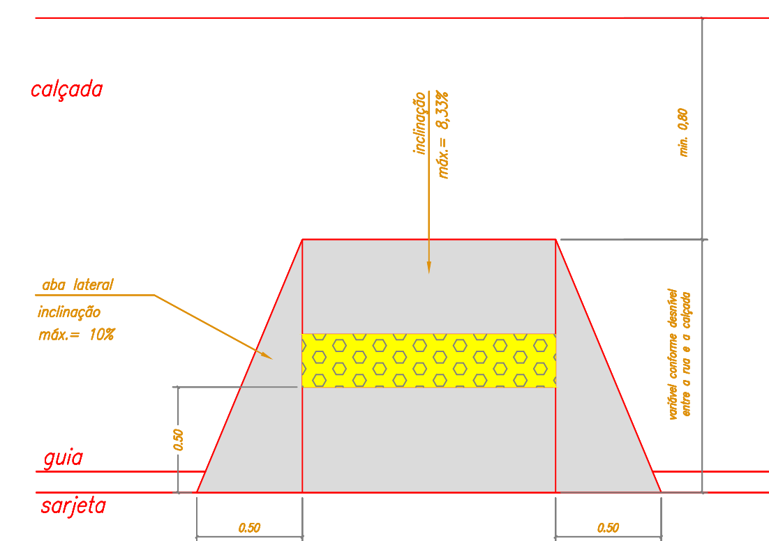
DETALHE DA RAMPA DE ACESSIBILIDADE ESC. 1:25
