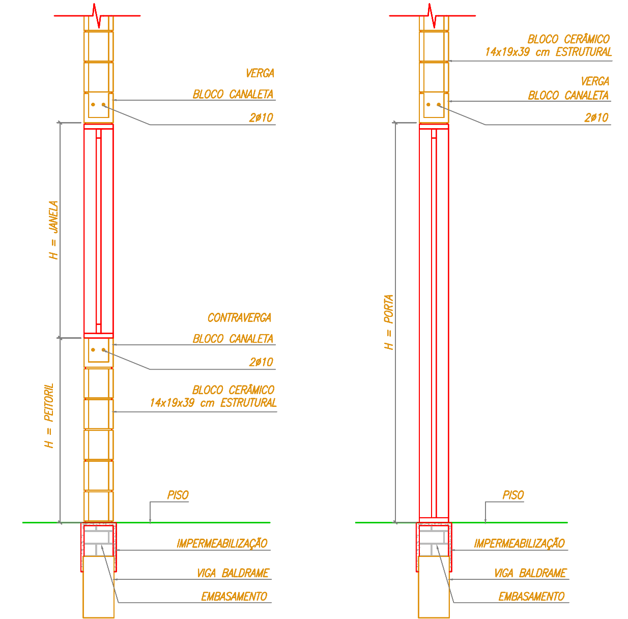
DETALHE DA ALVENARIA ESC. 1:25
