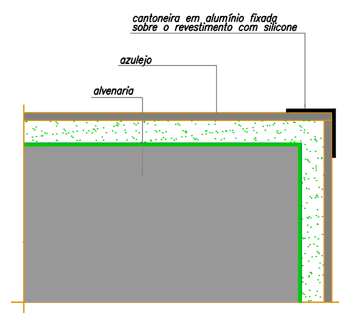
DETALHE DA CANTONEIRA SOBRE REVESTIMENTO CERÂMICO SEM ESCALA
