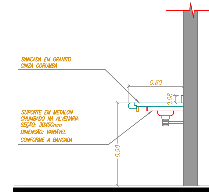
DETALHE DA BANCADELA DA COZINHA ESC. 1:25
