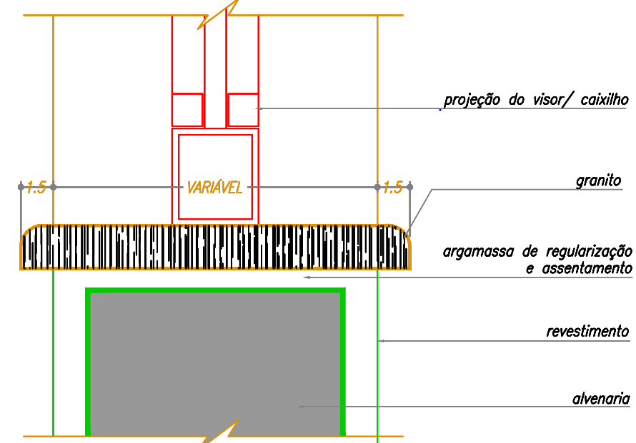
DETALHE DO RODAPÉ SEM ESCALA
