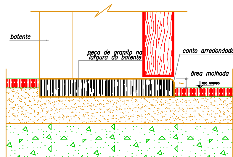
DETALHE DA SOLEIRAS PARA AS ÁREAS MOLHADAS SEM ESCALA
