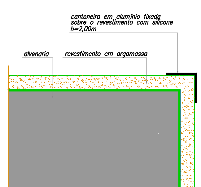
DETALHE DA CANTONEIRA SOBRE ARGAMASSA SEM ESCALA
