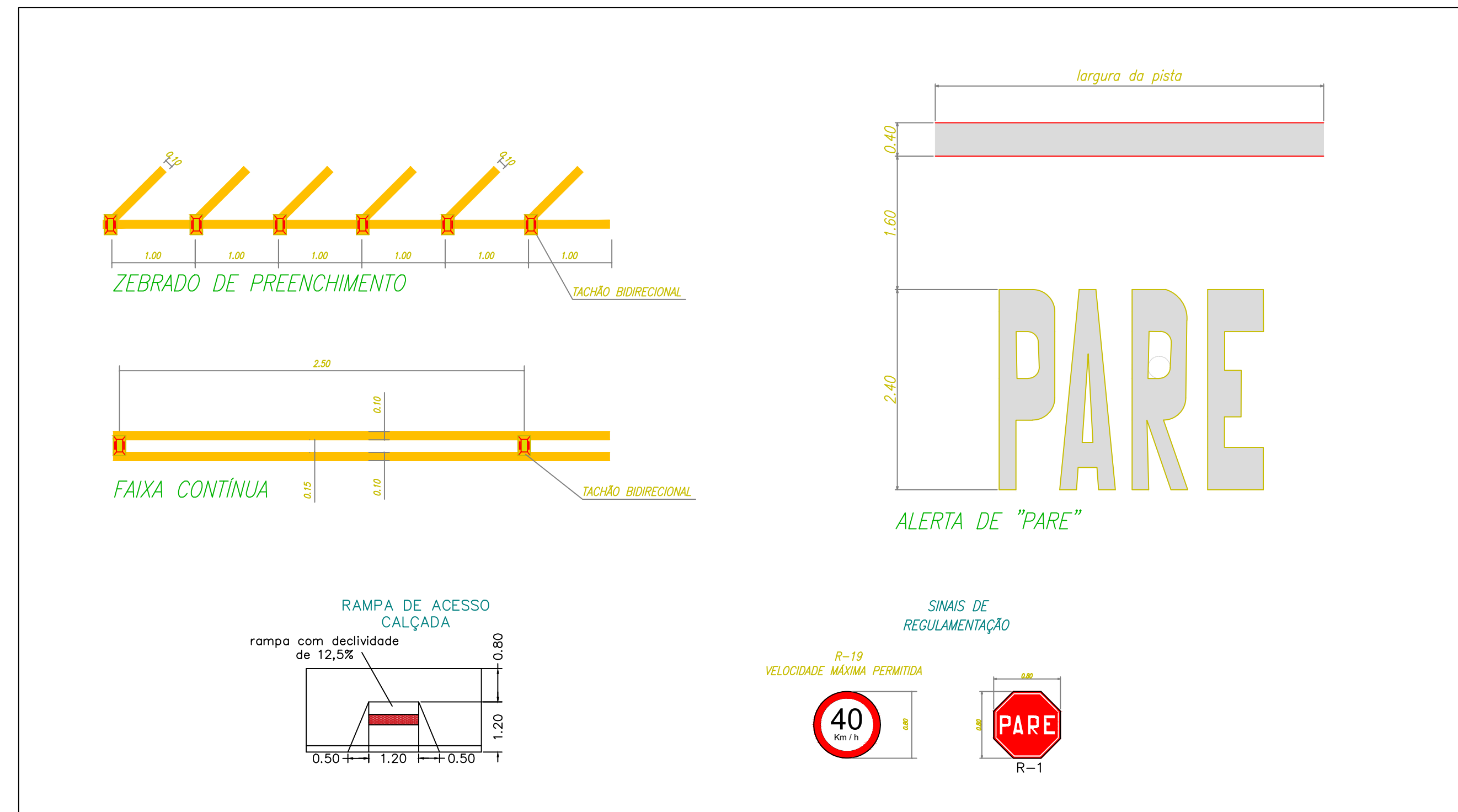
SINALIZAÇÃO VERTICAL E HORIZONTAL escala: 1:50
