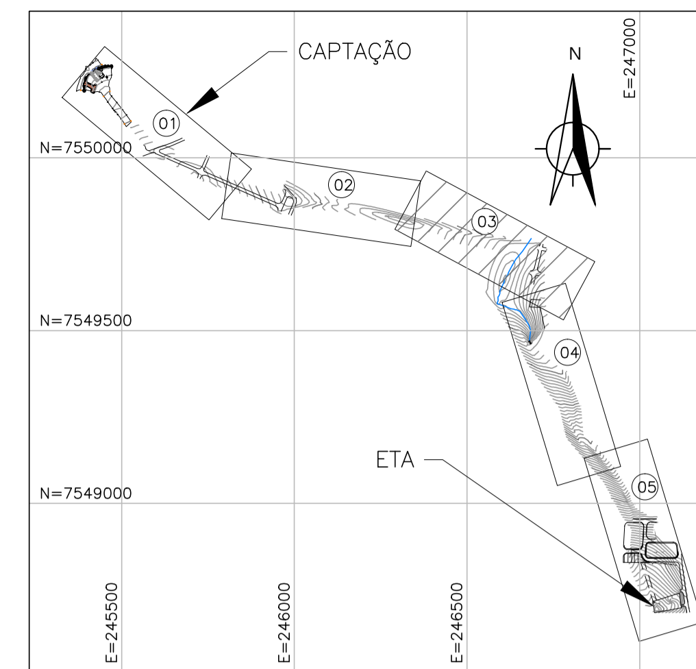
MAPA CHAVE ESC. 1:15000
