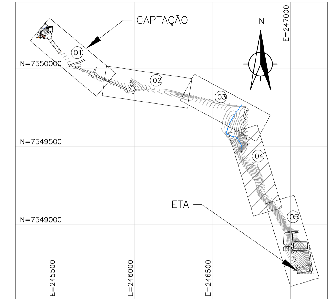
MAPA CHAVE ESC. 1:15000
