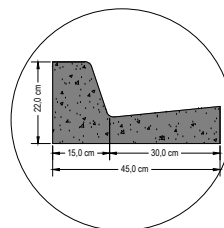
PERFIL DA GUIA SEM ESCALA
