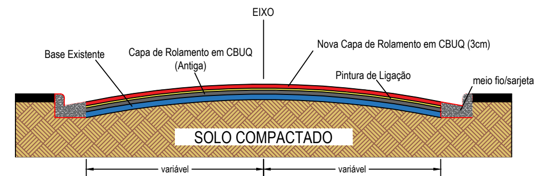
SEÇÃO TRANSVERSAL - RECAPEAMENTO ASFÁLTICO sem escala
